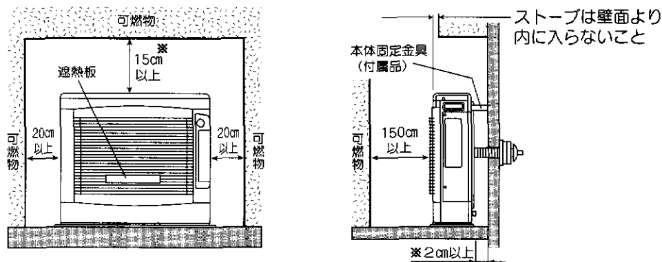
〔マントルピースなどに設置する場合のストーブ周囲寸法〕
