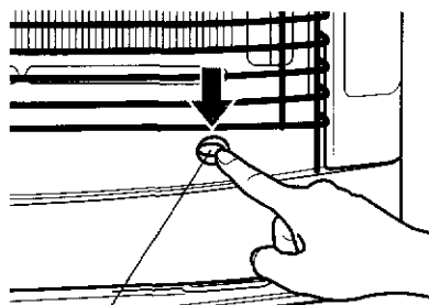
定油面器リセットボタン(赤色)
