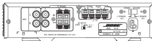
A 矢視図
